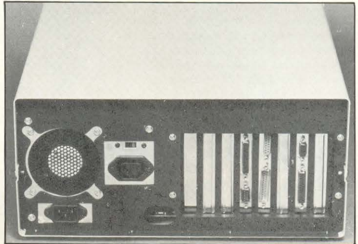
Η πίσω όψη του Betacom. Διακρίνονται οι θύρες των καρτών επέκτασης.
